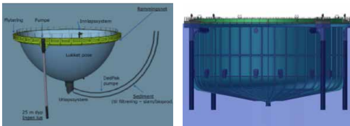
Figur 11. Principskiss över två olika typer av semislutna odlingssystem. (A) mjukt, flexibelt presserings-”skal” (Aquafuture). (B) Hårt, stål-förstärkt glasfiber skal med 40 m i diameter och 20 m djup 14 .
