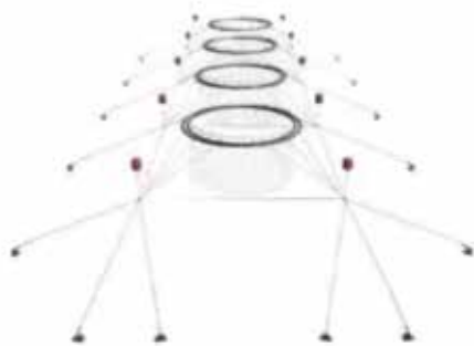
Figur 3. Principskisser över kassodlingar. Konstruktionen består av förankring, flytkonstruktion och en nätkasse.
